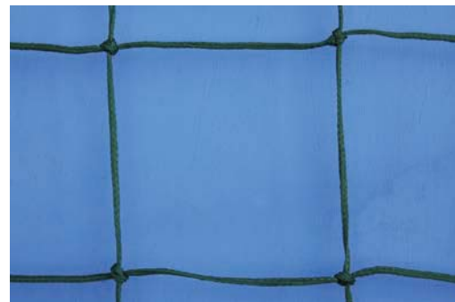
Art. 093.5 Rete protezione polietilene verde annodata maglia cm. 13x13 sp. mm.3,5 (per calcio e calcetto) Protection Net green polyethylene mesh 13x13 cm. knotted, thickness 3,5 mm.
